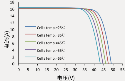
电流-电压曲线 (625W)
