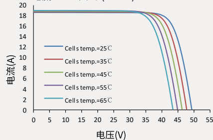
电流-电压曲线 (730W)
