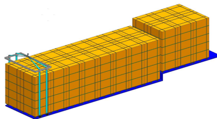
长边立式吊车卸货示意图
