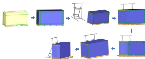
短边立式拆包步骤
