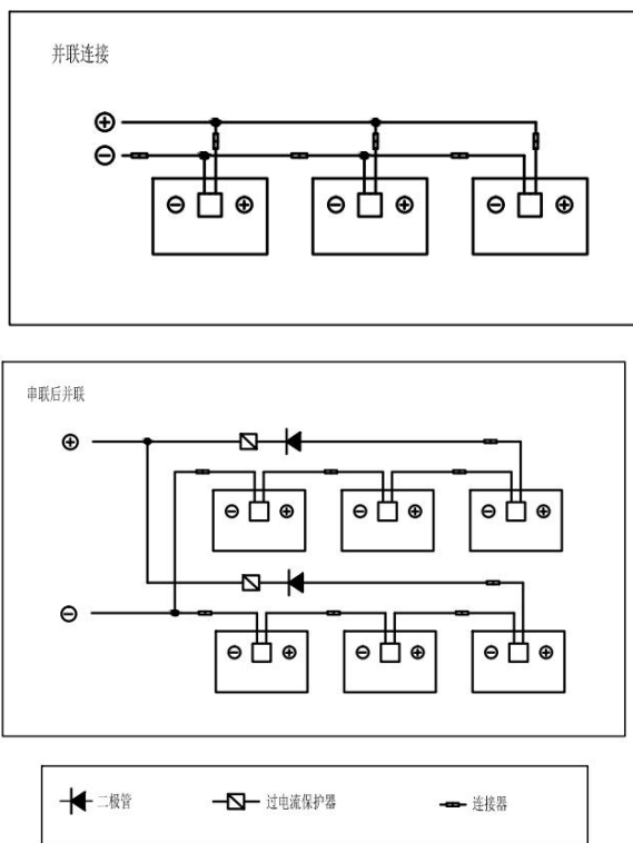
图 13 电连接示意图
