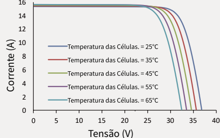
Corrente-Tensão (460W)
