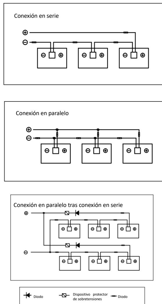
Fig. 13 Diagrama esquemático de conexión eléctrica
