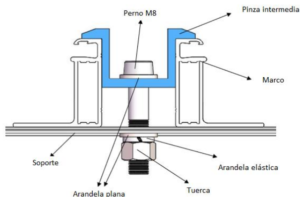
Fig. 12 Diagrama esquemático de instalación de pinza intermedia
