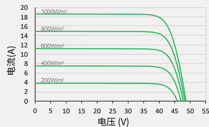
功率-电压曲线 (710W)
