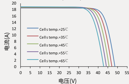
电流-电压曲线 (710W)
