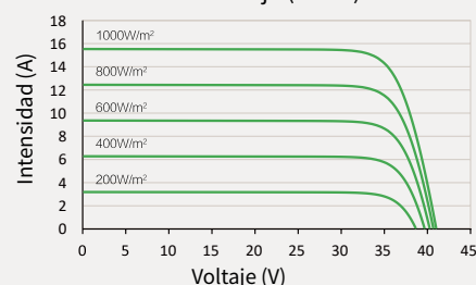
Potencia-voltaje (510W)
