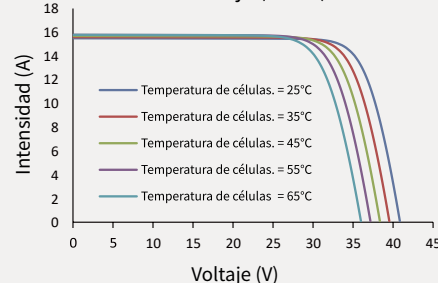
Intensidad-voltaje (510W)
