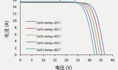
电流-电压曲线 (450W)
