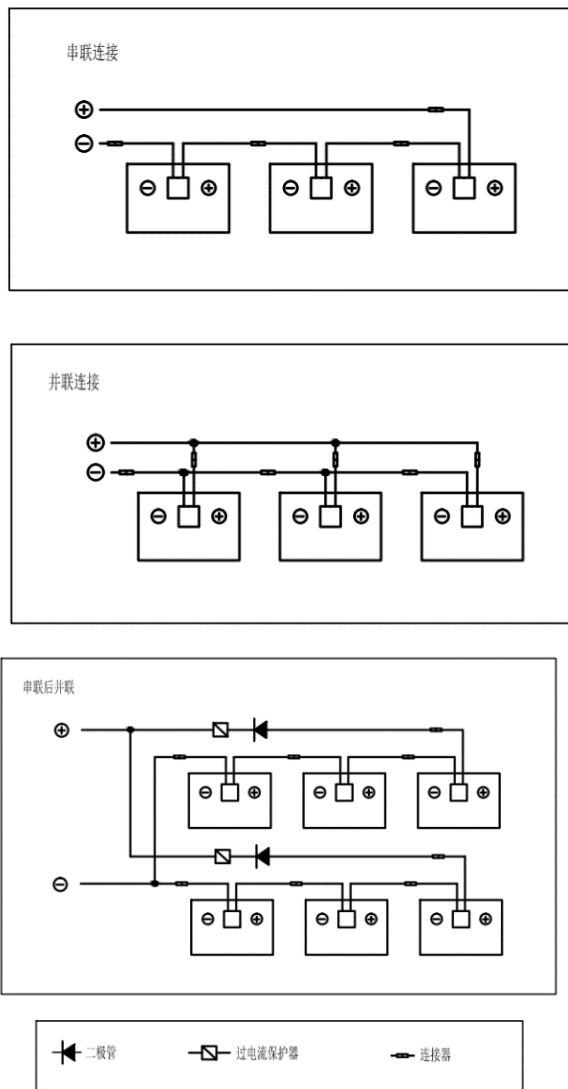
图 18 电联接示意图
