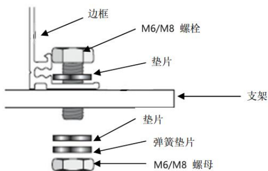
图10 螺栓安装过程示意图
