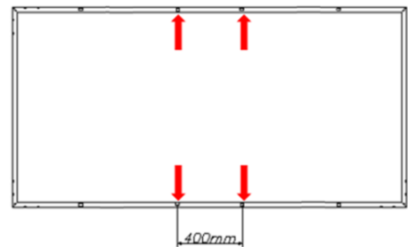
图 6 72cell 光伏组件内四孔螺栓安装
