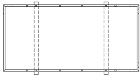
图 6 72cell 光伏组件内四孔螺栓安装
