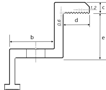
图 15 边压块横截面示意图
