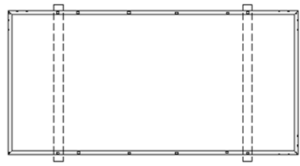
图 5 72cell 光伏组件外四孔螺栓安装
