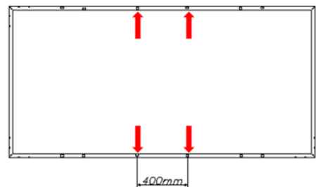
图 8 66cell 光伏组件 400mm 间距螺栓安装
