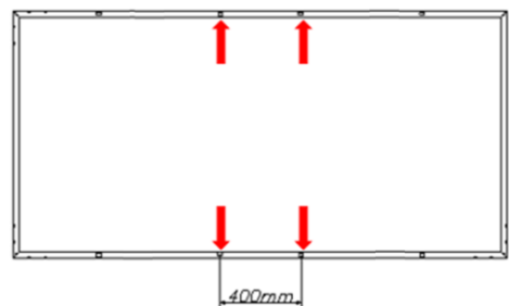
图 7 60cell 光伏组件 400mm 间距螺栓安装
