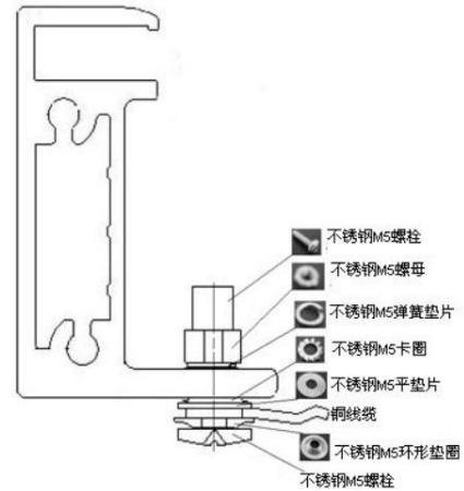
图 12 使用铜线缆将铝边框接地
