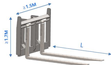
叉车门架：高 \geq 1.7M ，宽 \geq 1.5M ，
