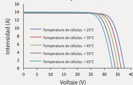
Intensidad-voltaje (410W)
